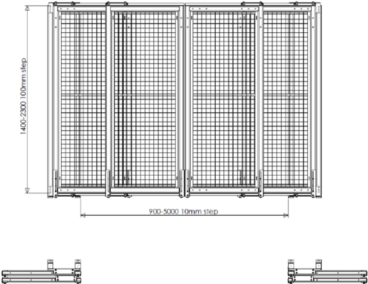
Porta doppia scorrevole a pavimento
