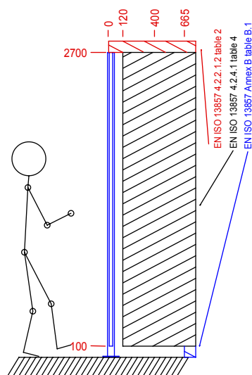
Distanza di sicurezza ad altezza 2700mm
