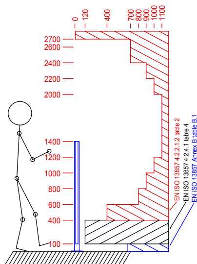
Distanza di sicurezza ad altezza 1400mm
