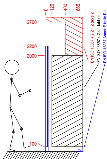
Distanza di sicurezza ad altezza 2200mm
