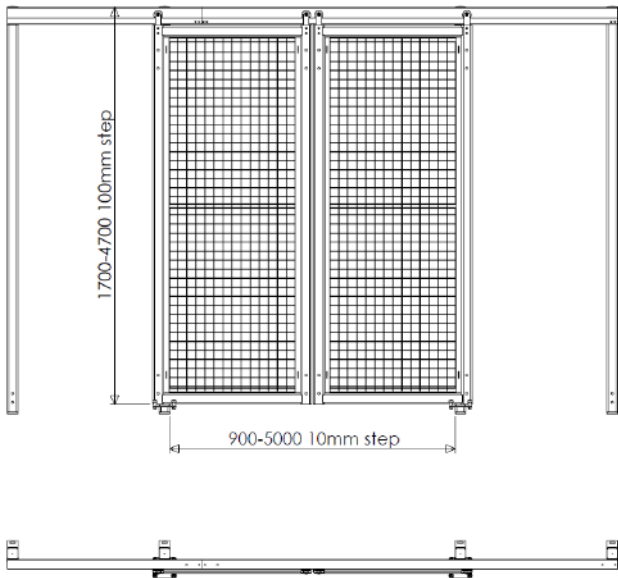
Porta scorrevole doppia con binario superiore
